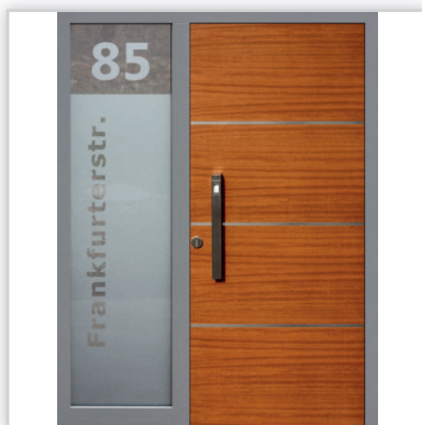
Drzwi wejściowe zewnętrzne model 490,20 z opcjonalną dostawką boczną i czytnikiem linii papilarnych wbudowanym w antabę. Grubość [mm]: 82. Wysokość ościeżnicy 209. Szerokość całej zabudowy od 140 do 250 cm. Wyposażenie: zamek listwowy klasy „C” na dwie wkładki, 4 blokady antywłamaniowe. Szklenie: pakiet 3 szybowy z szybą niskoemisyjną P1. Materiał: klejone warstwowo drewno mahoń-meranti. Ocieplenie [mm]: 58. Współczynnik przenikania ciepła U_d [W/(m 2 K)]: 0,7. Gwarancja: 4 lata.
